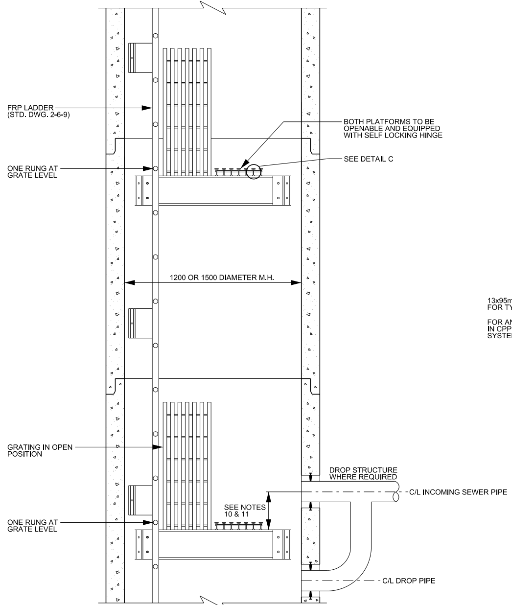
SECTION A-A
